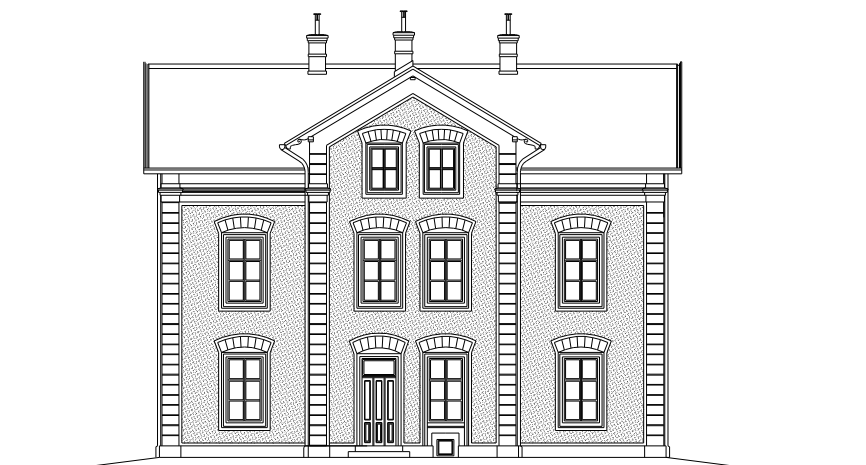
VÁROS FELŐLI HOMLOKZAT
