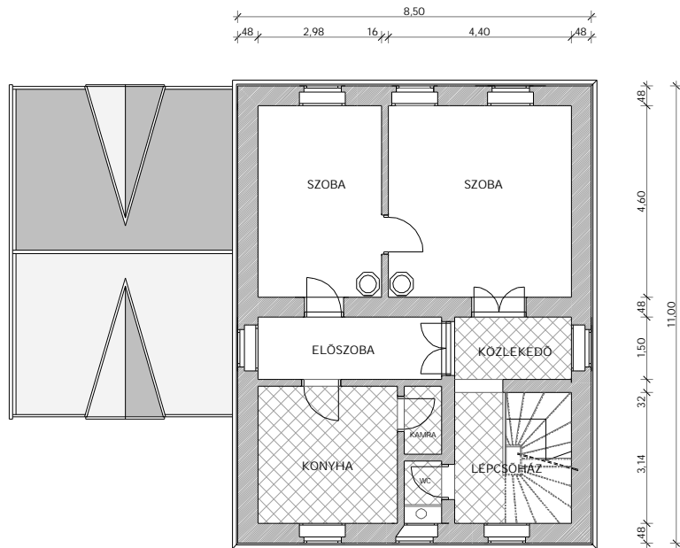
EMELETI ALAPRAJZ
