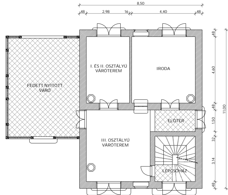
FÖLDSZINTI ALAPRAJZ
