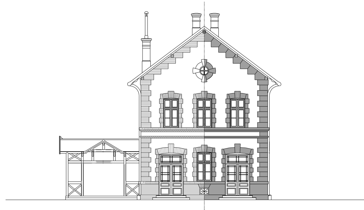
PÁLYA FELŐLI HOMLOKZAT
