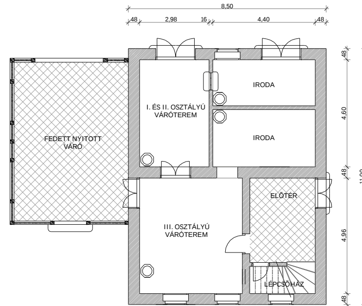
ALAPRAJZ
