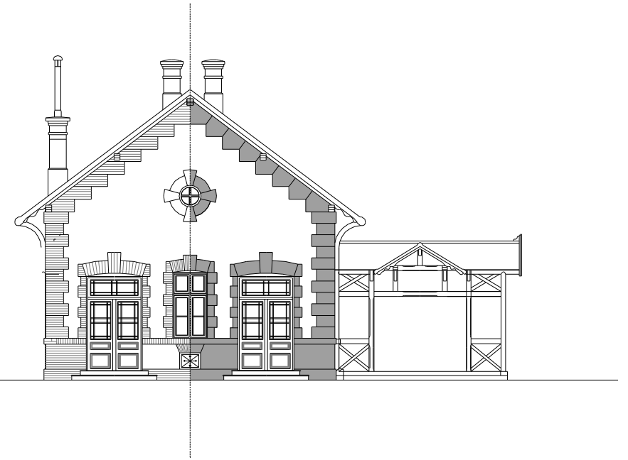
PÁLYA FELŐLI HOMLOKZAT
